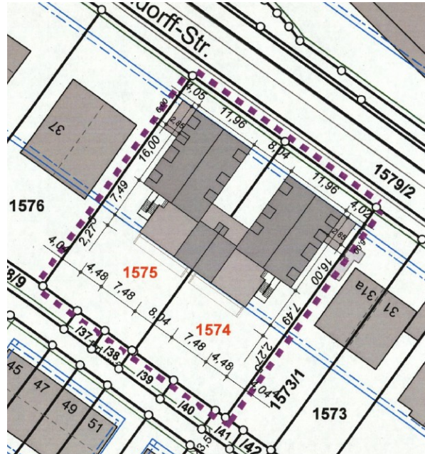
Auszug Lageplan
