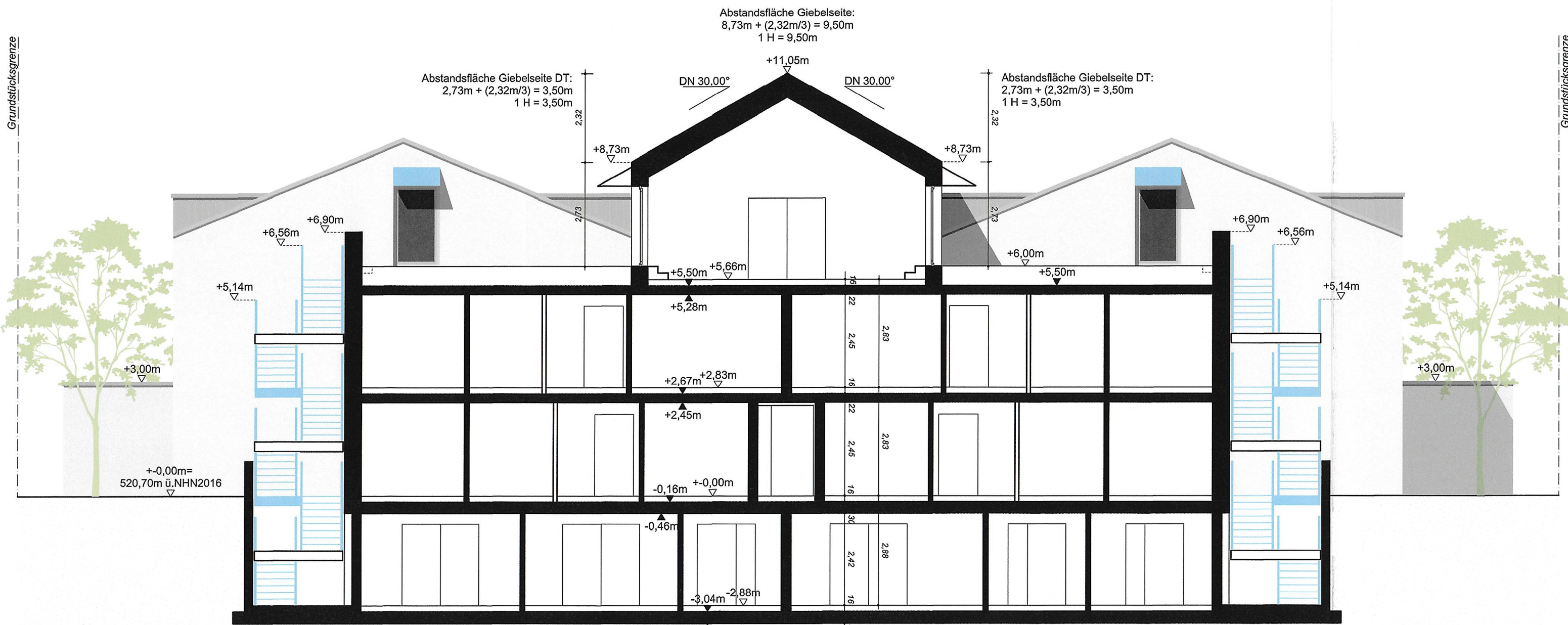
Schnitt B-B
