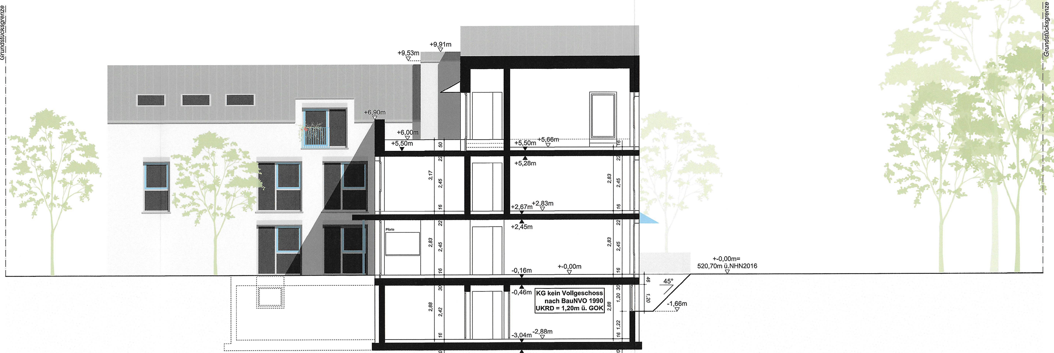
Schnitt C-C
